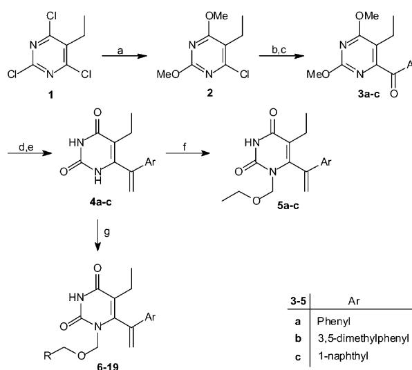
Scheme 1. (a) Ref 18; (b) ArCH 2 CN, NaH, DMF; (c) NaH, O 2 , DMF, 66–93% (one-pot synthesis); (d) CH 3 MgBr, THF; (e) HCl (aq), 69–86% (two steps); (f) BSA, CH 3 CH 2 OCH 2 Cl, CHCl 3 , 24–48%; (g) BSA, TMS-triflate, RCH 2 OCH 2 OCH 2 R, CH 3 CN, 10–99%.
